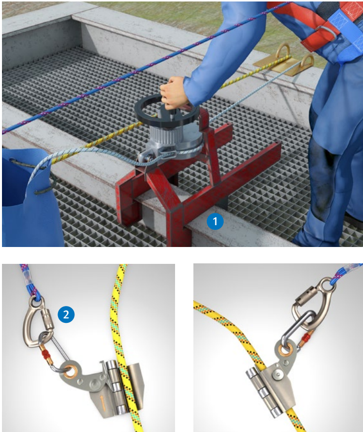
Abb. 6 Einsatz des Rettungsgeräts und einer Seilklemme
