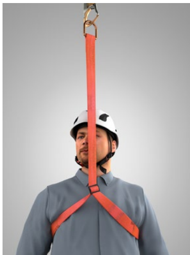
Abb. 11 Rettungsschleife der Klasse A
